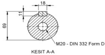
KESİT A-A
